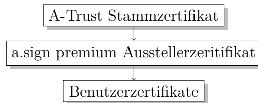
Abbildung 1: Zertifikatshierarchie
